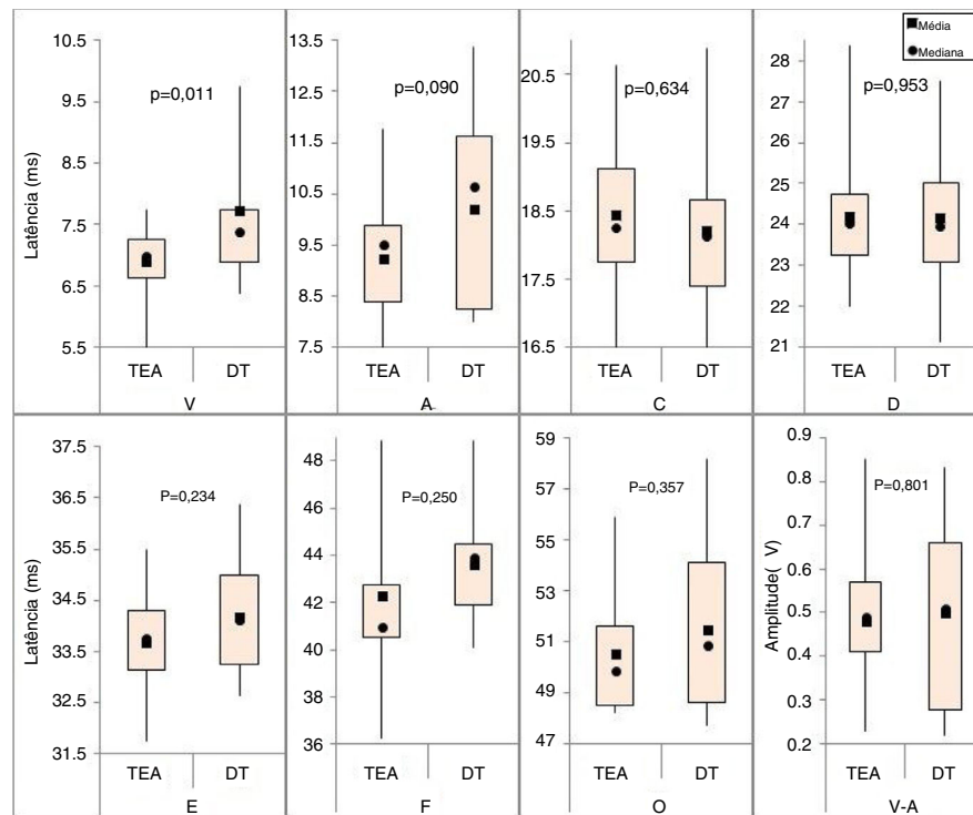
Figura 3 Medidas descritivas das latências das ondas V, A, C, D, E, F e O e da amplitude V-A dos PEATEs com estímulos de fala, por grupo e ouvido. TEA, Transtornos do Espectro do Autismo; DT, Desenvolvimento Típico; ms, milissegundos; \mu V, microvolts.
